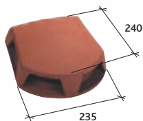
Klobouk prostupové tašky Ø 120 a Ø 150 (130 cm 2 ) Réf. 1000
