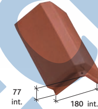
Hřebenáč (3 ks/bm) Réf. 710
