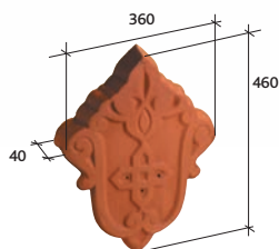
Ukončení univerzální okrajové tašky Réf. 1083
