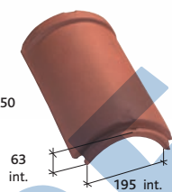
Hřebenáč (2,5 ks/bm) Réf. 702
