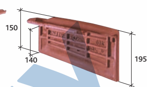
Okrajová taška pravá (4 ks/bm) Réf. 301.41
