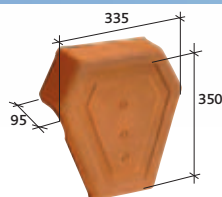
Ukončení hřebenáče univerzální Réf. 1080
