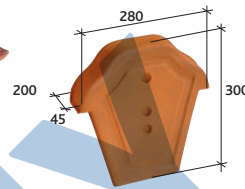
Ukončení hřebenáče Losangée Réf. 809
