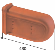
Ukončení univerzální okrajové tašky pravé Réf. 1070
