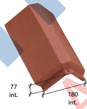
Hřebenáč (3 ks / bm) Réf. 710
