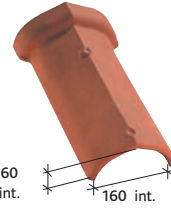
Hřebenáč nároží (2,5 ks / bm) Réf. 758
