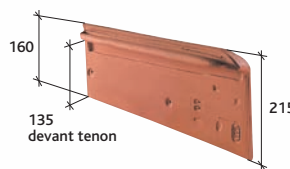
Pravá okrajová taška (2,7 ks / bm při laťování 376 mm) Réf. 215.41
