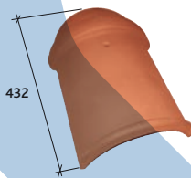
Koncový hřebenáč Réf. 869
