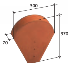
Ukončení hřebenáče velké Réf. 804
