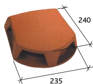
Klobouk prostupové tašky Ø 120 a Ø 150 (130 cm 2 ) Réf. 1000
