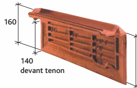
Pravá okrajová taška (2,7 ks / bm při laťování 390 mm) Réf. 200.41
