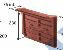
Univerzální okrajová taška (3 ks / bm) Réf. 1051
