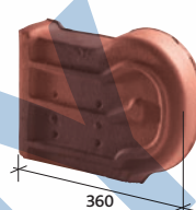
Ukončení univerzální okrajové tašky levé Réf. 1072
