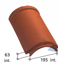
Hřebenáč (2,5 ks / bm) Réf. 702
