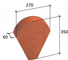
Ukončení hřebenáče malé Réf. 803
