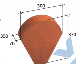
Ukončení hřebenače velké Réf. 804
