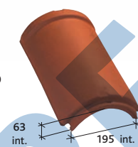
Hřebenač (2,5 ks / bm) Réf. 702
