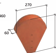
Ukončení hřebenače malé Réf. 803
