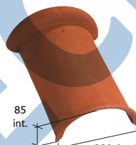
Hřebenač půlkruhový (2,5 ks / bm) Réf. 715
