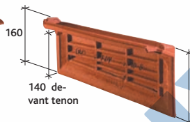
Pravá okrajová taška (2,6 ks / bm při laťování 390 mm) Réf. 202.41
