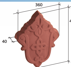
Ukončení univerzální okrajové tašky Réf. 1083
