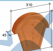
Ukončení hřebenáče Réf. 807
