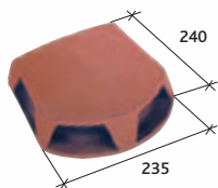
Klobouk prostupové tašky Ø 120 a Ø 150 (130 cm²) Réf. 1000
