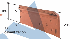
Individuální okrajová taška pravá Réf. 215.41
