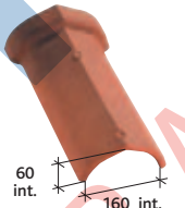
Hřebenáč (2,5 ks / bm) Réf. 758
