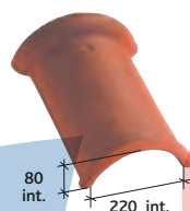
Hřebenáč 1/2 kruhový (2,5 ks/ml) Réf. 717
