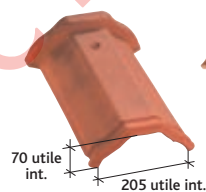
Hřebenáč Losangée (2,5 ks / bm) Réf. 716
