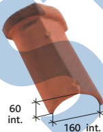
Hřebenáč nároží (2,5 ks / bm) Réf. 758
