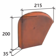
Ukončení pultového hřebenáče levé Réf. 806
