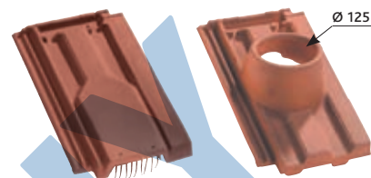
Větrací taška větrací otvor 33 cm 2 Réf. 215.20
