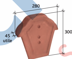
Ukončení hřebenáče Losangée Réf. 809
