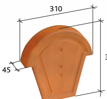
Ukončení 1/2 kruhového hřebenáče Réf. 807
