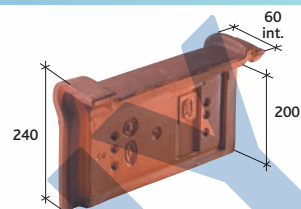
Individuální okrajová taška (3 ks / bm) Réf. 1050
