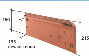
Pravá okrajová taška (2,8 ks / bm při laťování 364 mm) Réf. 215.41
