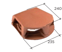
Dvousekční klobouk Ø 126 a Ø 160 (větrací průřez 259 cm 2 ) (v souladu s VMC) Ref. 100 9
