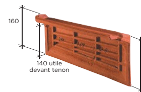
Individuální okrajová taška DELTA 10 Ste Foy Pravá (Droite) - Ref. 202.41 Levá (Gauche) - Ref. 202.42
