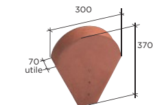
ukončení hřebene hůdké, 1/2kolaté Ref. 804
