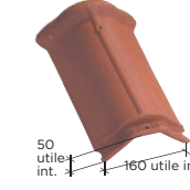
hřebenáč reliéf (3 na ml) Ref. 706 Háček F6 pro hřebenovou 1/2 kulatou tašku - malý, se zámkem Ref. CRP700/706
