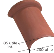
Hřebenáč 1/2kruhový (2,5 na ml) Ref. 715 Háček F5 pro hřebenovou tašku s listou a se zámkem - Ref. CRP715
